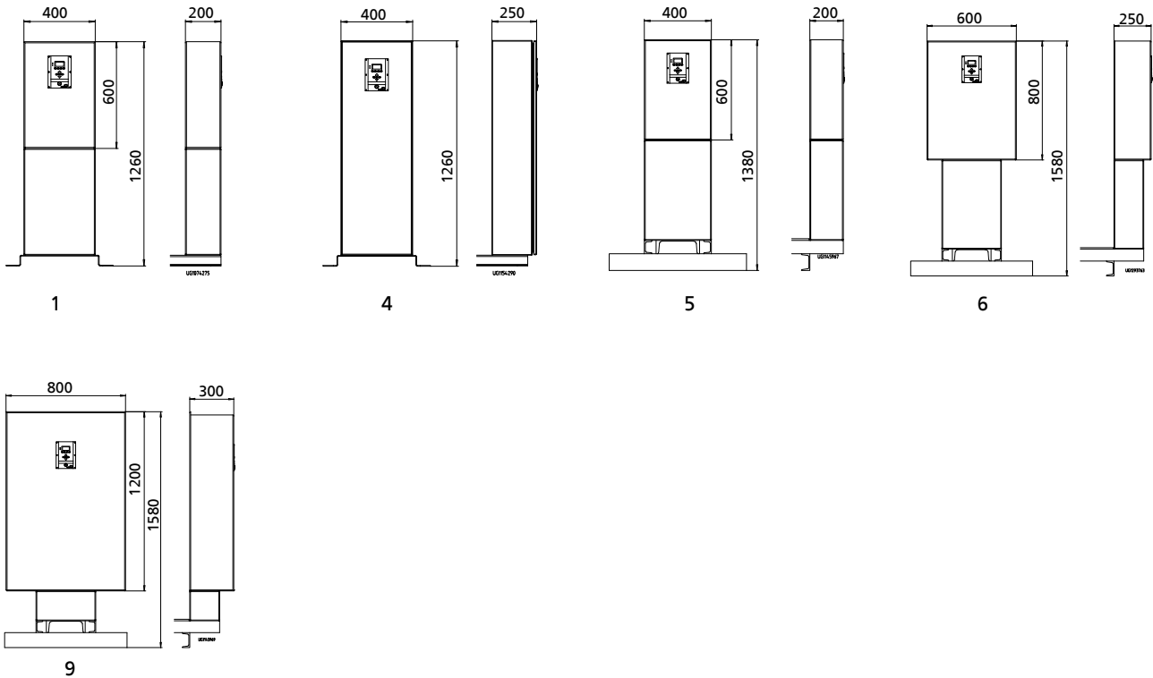
Dimensions armoire de commande Hyamat SVP [mm]
